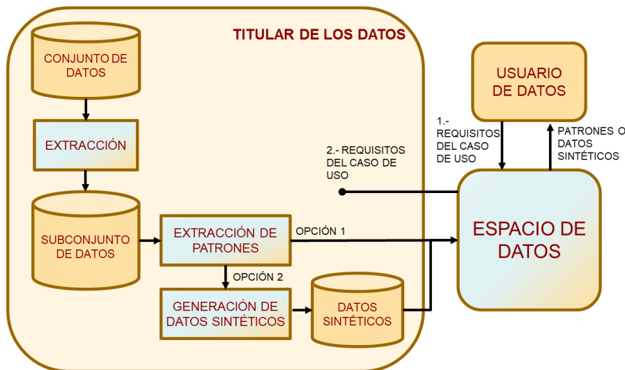
Figura 20: Esquema de la arquitectura para el caso de uso de puesta a disposición datos sintéticos
