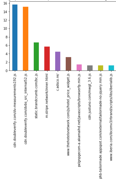
Scripts canvas fingerprint detectados por llamadas a (toDataURL o getImageData) y fillText
