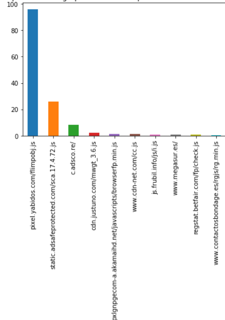
Scripts webRTC fingerprint detectados por llamadas a onicecandidate
