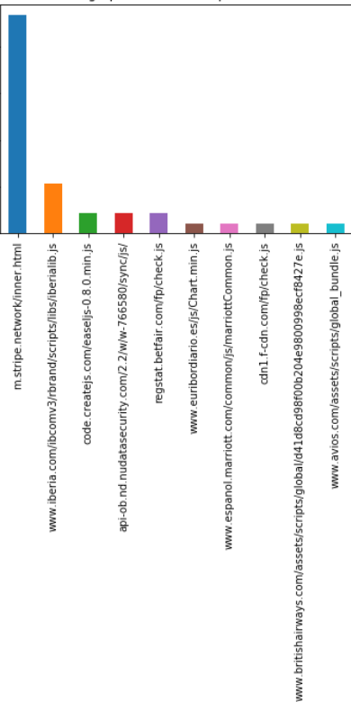
Scripts canvas font fingerprint detectados por llamadas a measureText
